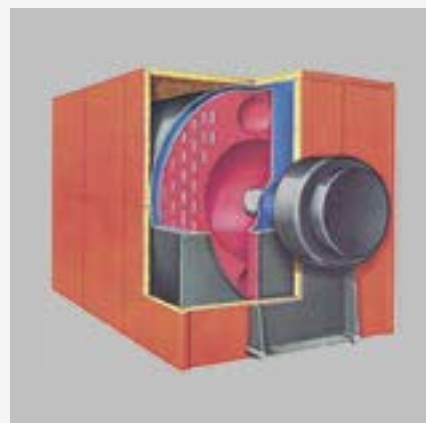
Turbomat-L – водогрейный /паровой котел 1869-9300 кВт
