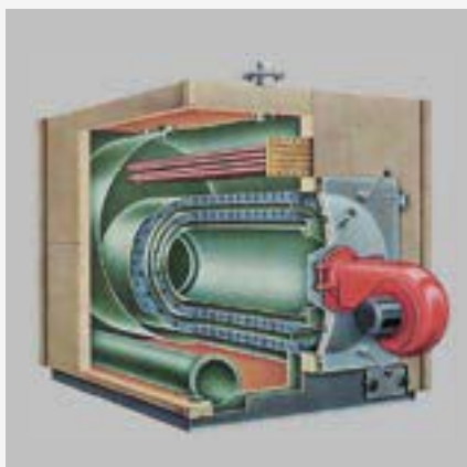
Turbomat – водогрейный/паровой котел 140-4652 кВт
